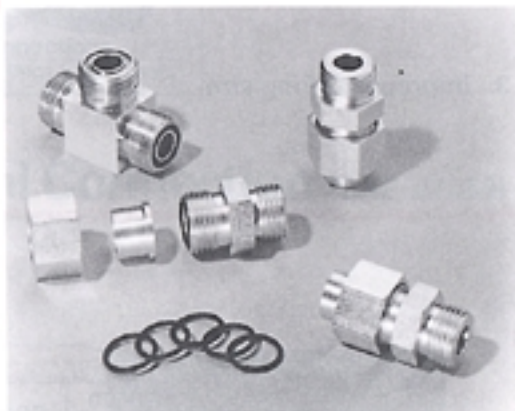
Aeroquip ORS connections
