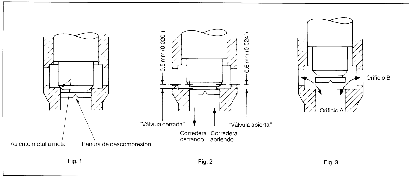
Fig. 1: Válvula completamente cerrada por la presión hidráulica piloto y/o el muelle. La corredera está completamente ajustada dentro de la camisa.
