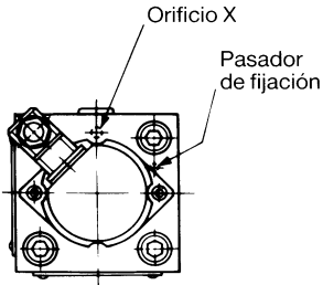
Vista mostrando la orientación del interruptor y del enchufe en CVU-16-SWD-B29-**-10
