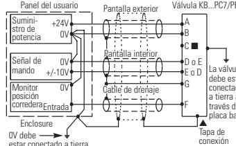
Figura 1 Conexiones de cableado para válvulas con amplificador incorporado
