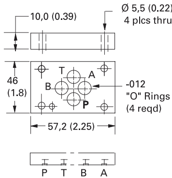
Blanking Plate 02-185274
