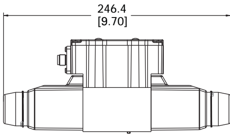
DG4V-3-* C/N-H -*M-PM4*S-***7-70
