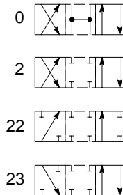
DG4V-5-*A Ventile
