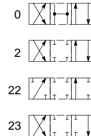
DG4V-5-*AL Ventile
